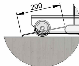
DETAIL B // Rampe dimensioner (mm) SCALE 1 : 10
