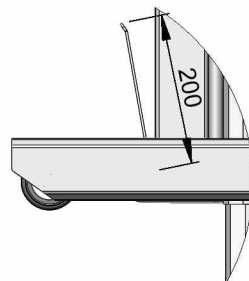
DETAIL C // Rampe dimensioner (mm) SCALE 1 : 10
