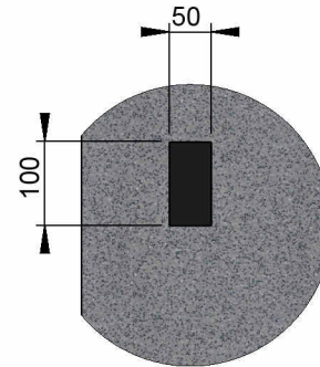
DETAIL D SCALE 1 : 10 Aktuatorposition / fodaftrek
